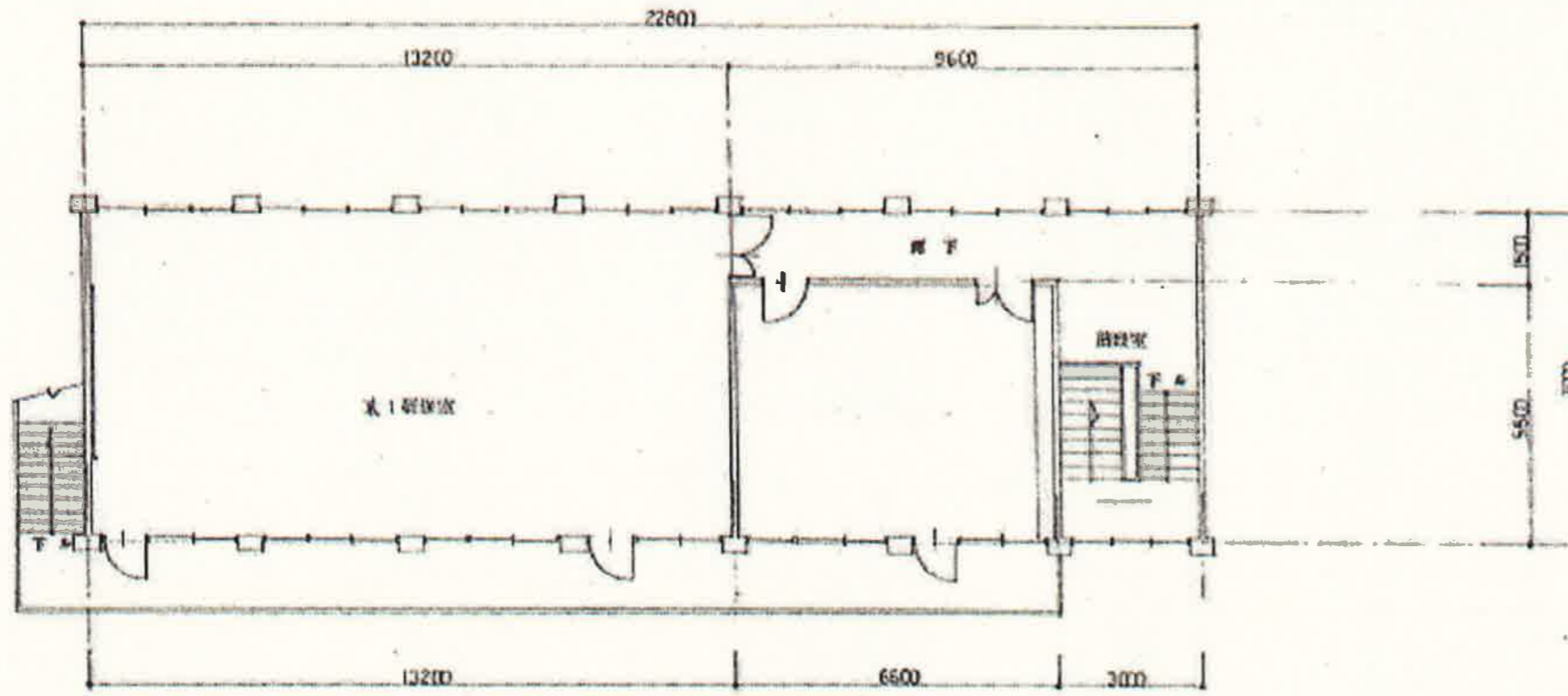
2階平面図
