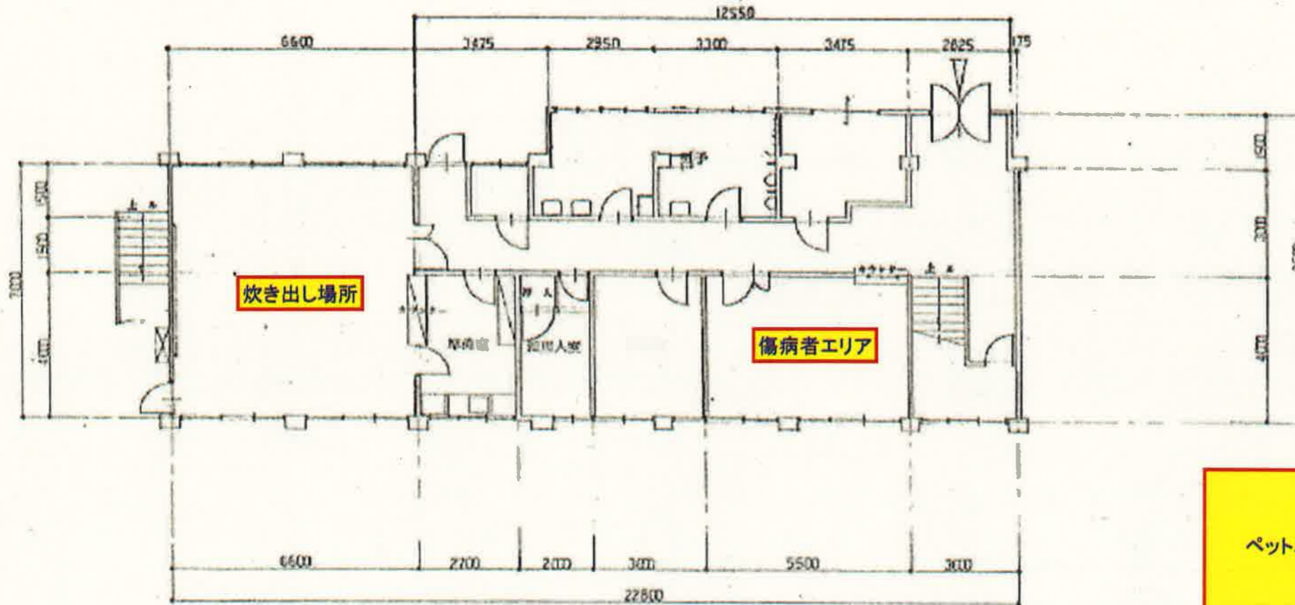
2階平面図
