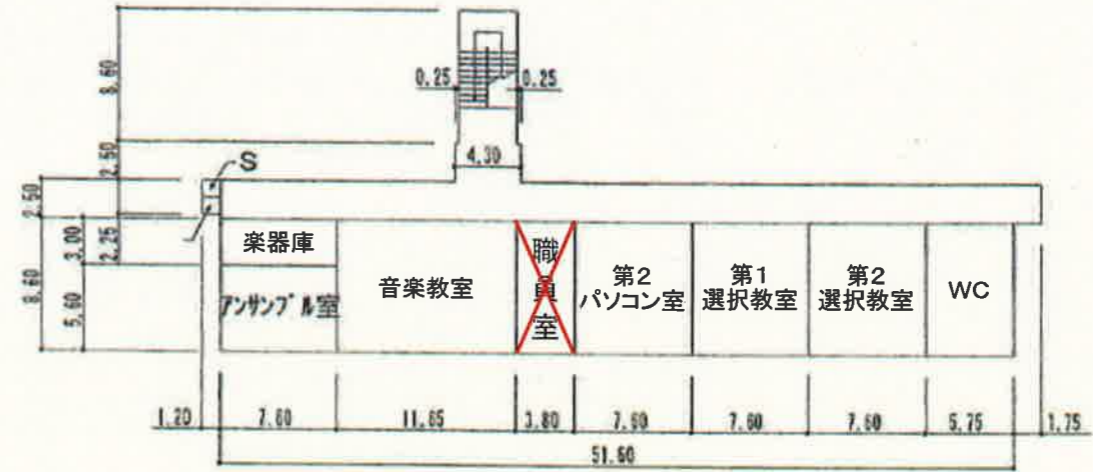
3階
