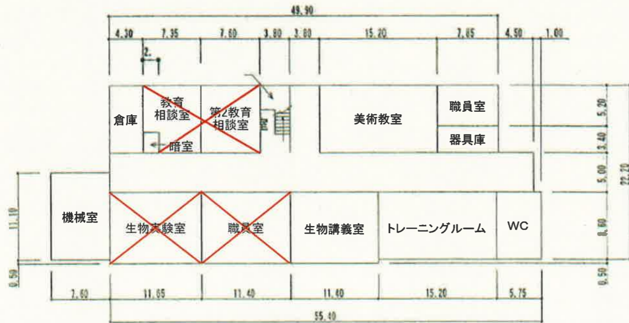
1階
