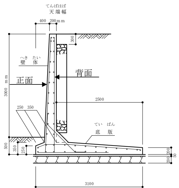
鉄筋コンクリートL型擁壁の例
