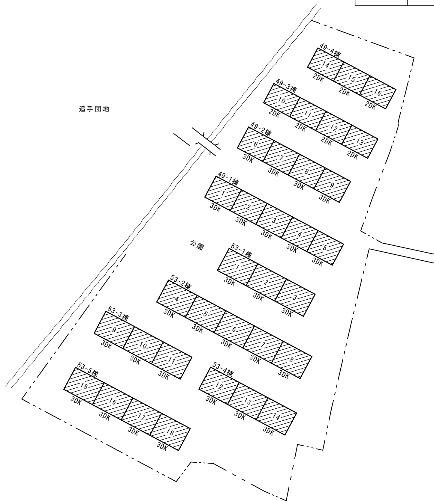
新町団地 配置図
