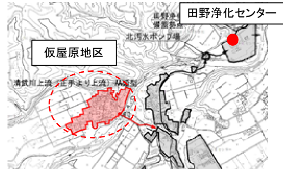
(田野町仮屋原地区の公共下水道接続位置図)
