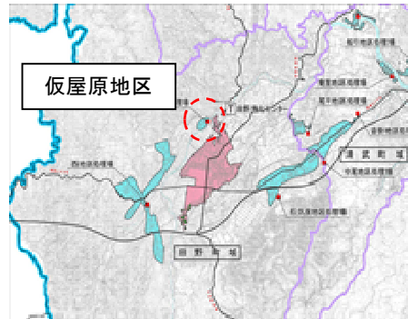
(田野町仮屋原地区の農業集落排水施設の位置図)
