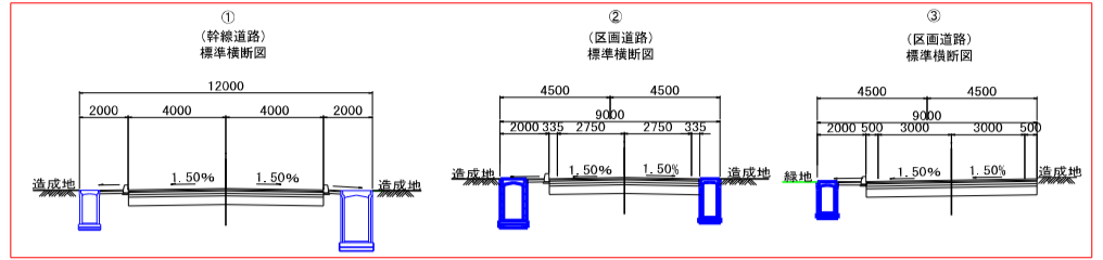
道路横断面図
