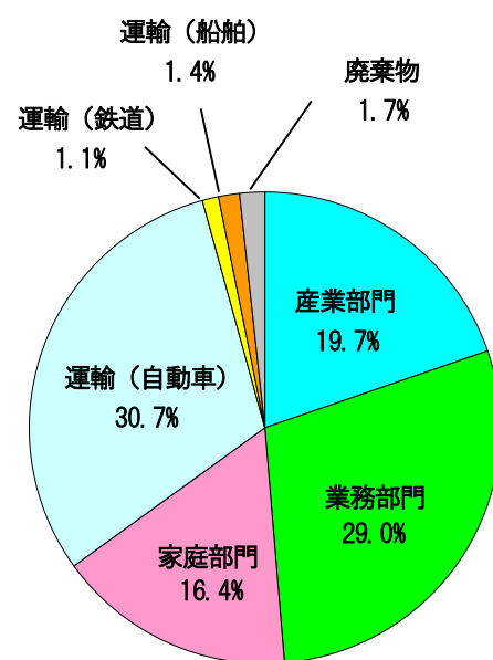
二酸化炭素(CO 2 )の部門別排出割合(令和元年度)
