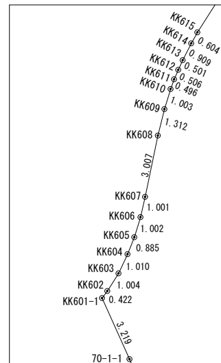
拡大図A 1/250
