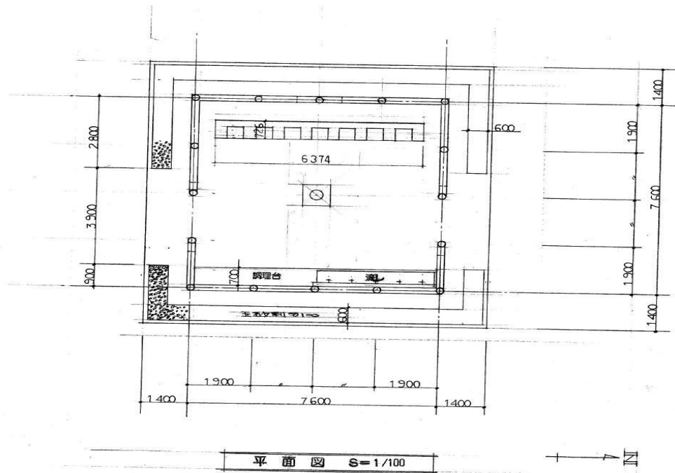
炊飯棟見取り図
