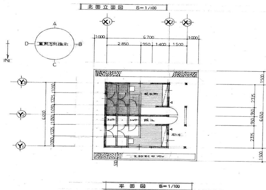
シャワー棟見取り図
