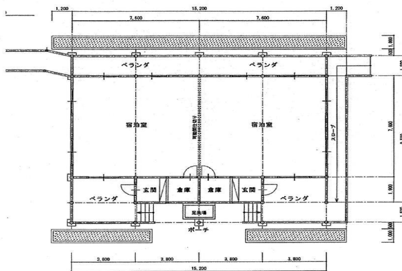
ログハウス A棟 平面図
