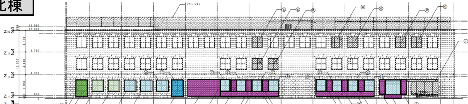
家屋立面図・平面図
