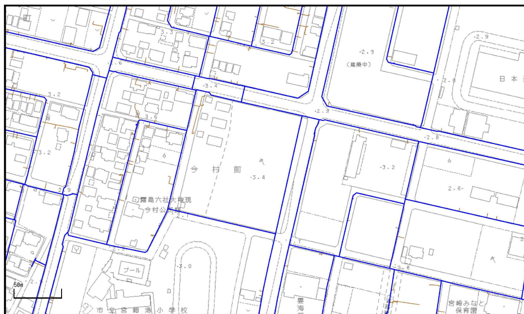
宮崎市上水道参考図
