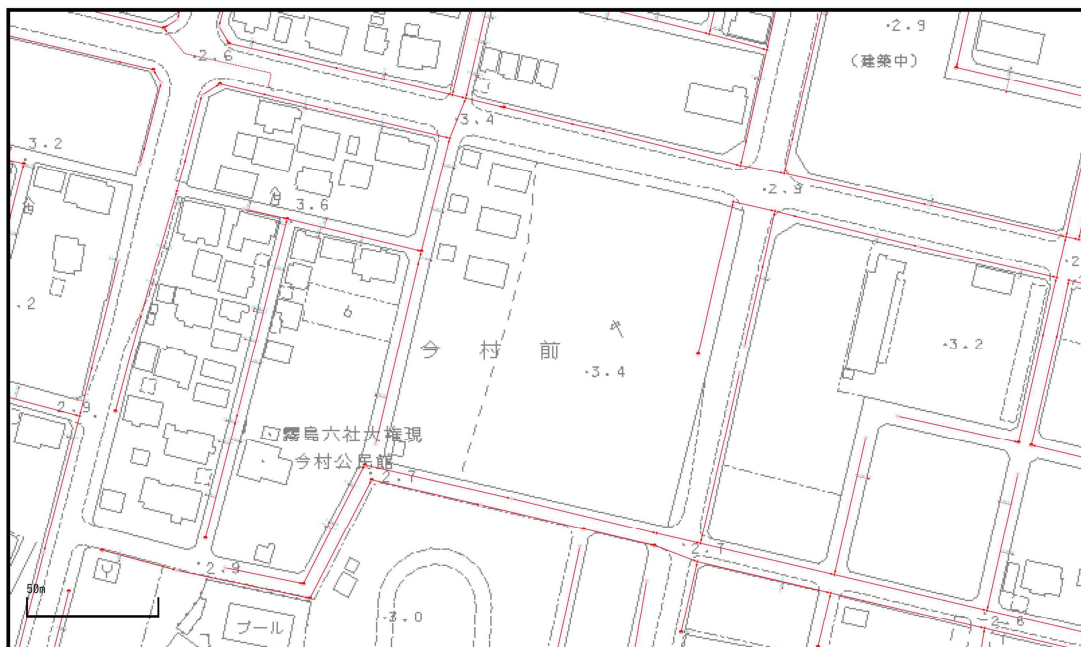
宮崎市下水道参考図
