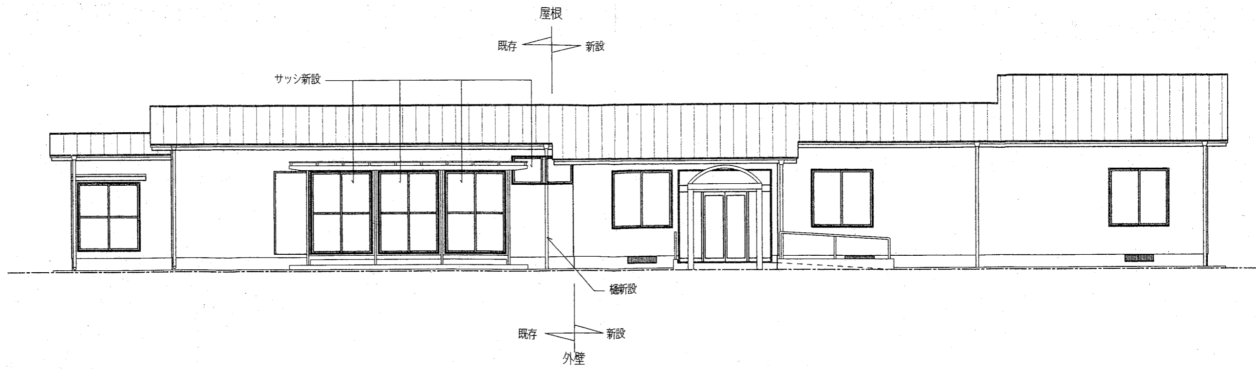
東立面図 1/100
