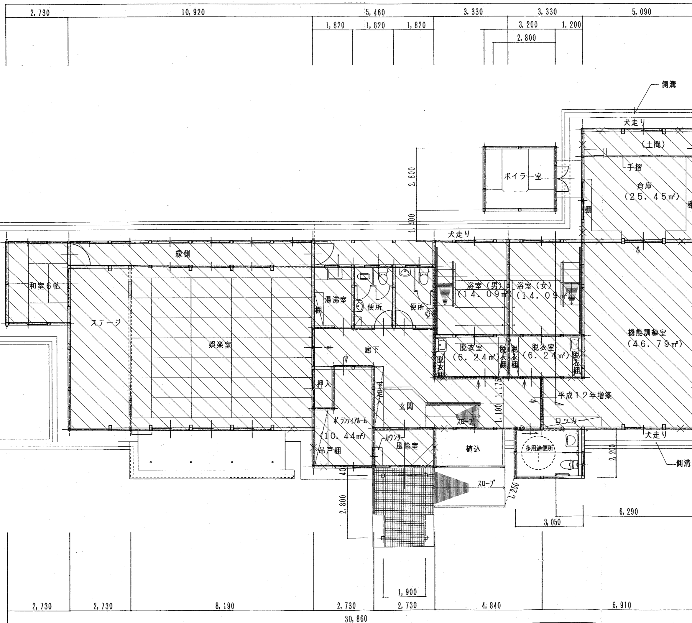
増築後平面図
